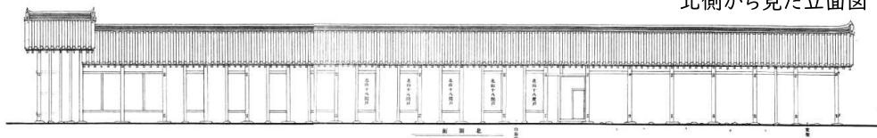
北側から見た立面図
