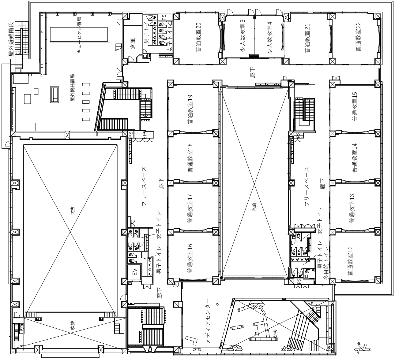
3 階平面図
