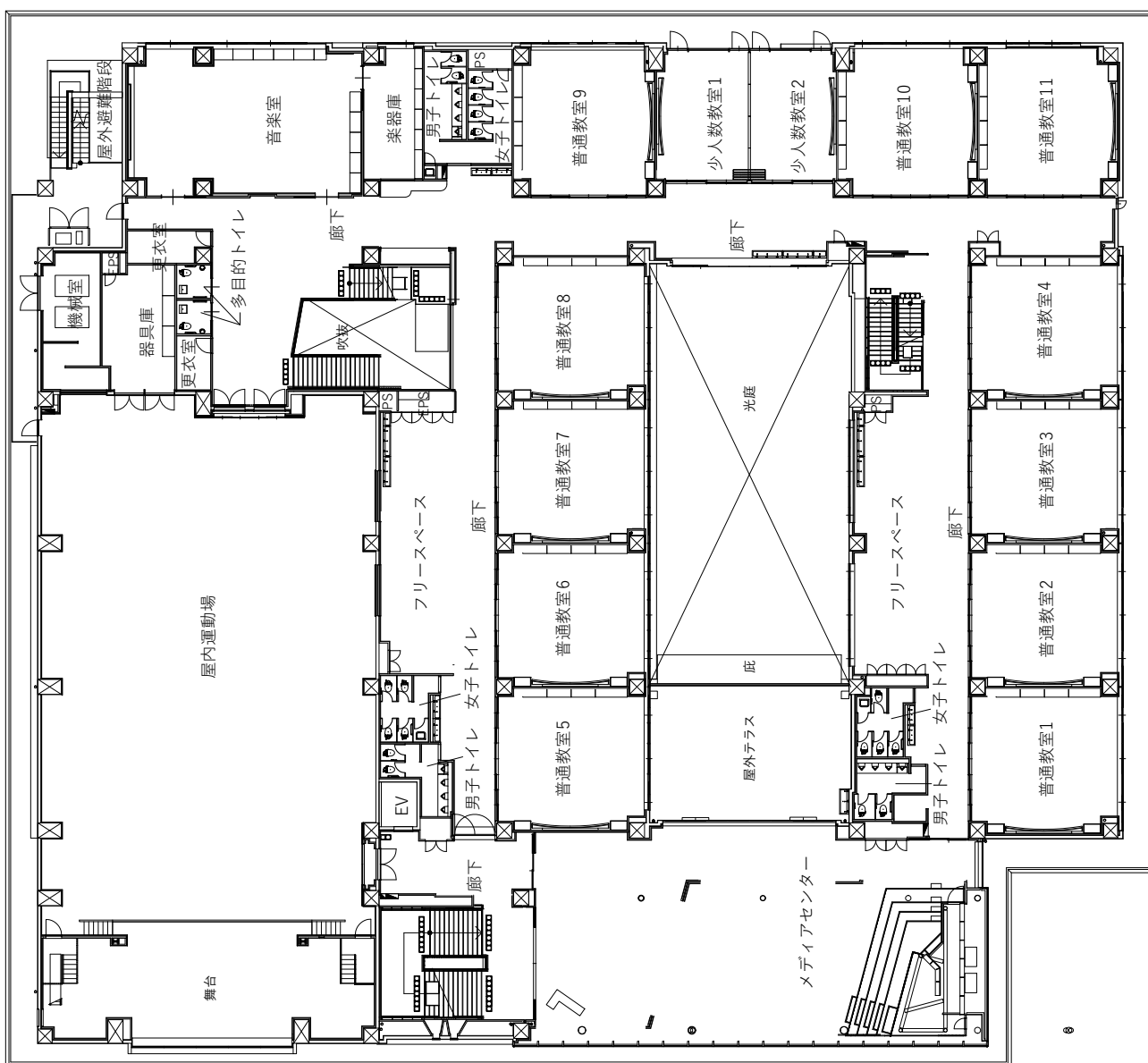
2階平面図
