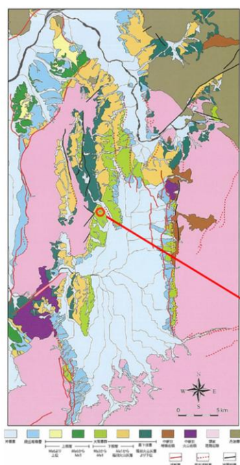
口絵2 奈良盆地の地質
